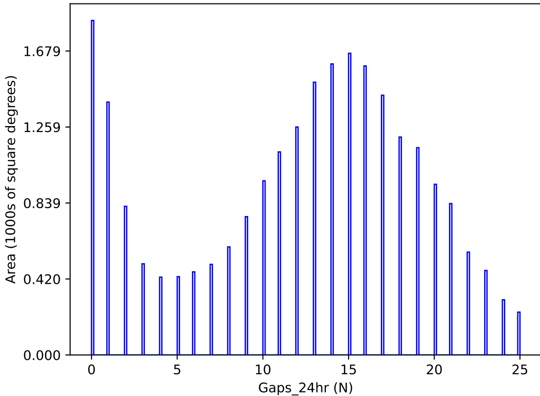
weather_cloudso31v3.4_10yrs y band: Gaps_24hr
