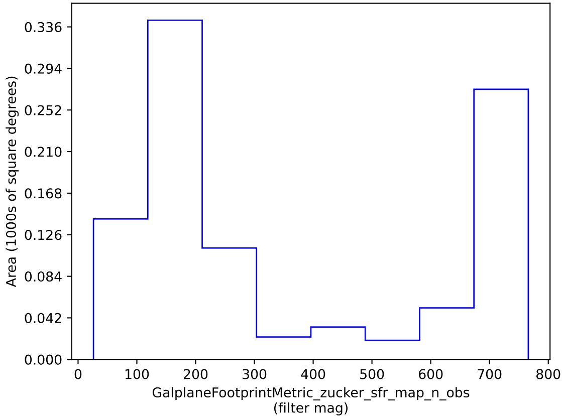
weather_cloudso31v3.4_10yrs : GalplaneFootprintMetric_zucker_sfr_map_n_obs
