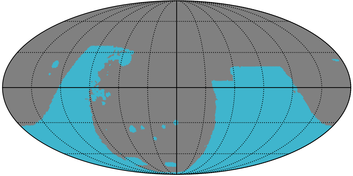
weather_cloudso31v3.4_10yrs : GalplaneFootprintMetric_combined_map_Tau_2_0
