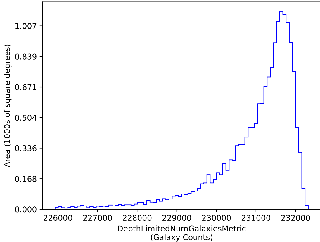
weather_cloudso31v3.4_10yrs i band galaxies non-DD: DepthLimitedNumGalaxiesMetric
