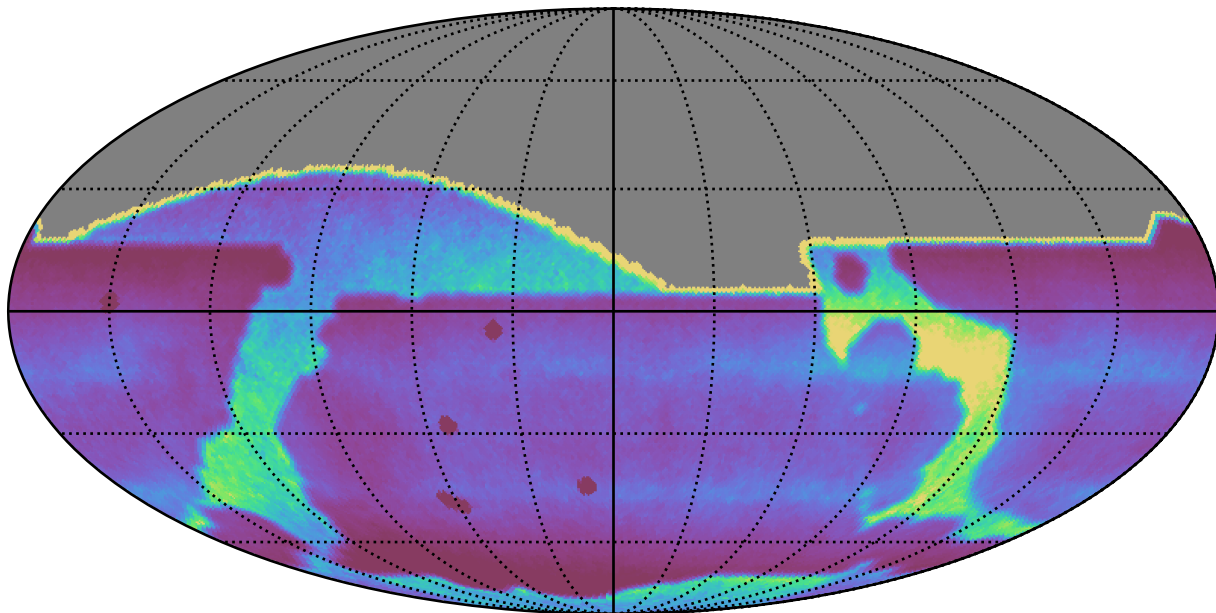
weather_cloudso31v3.4_10yrs : DCRprecision
