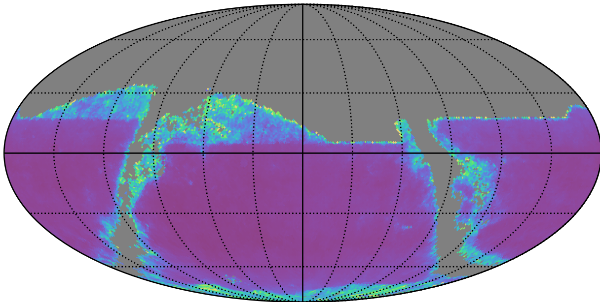
weather_cloudso31v3.4_10yrs z band: AGN SF_uncert
