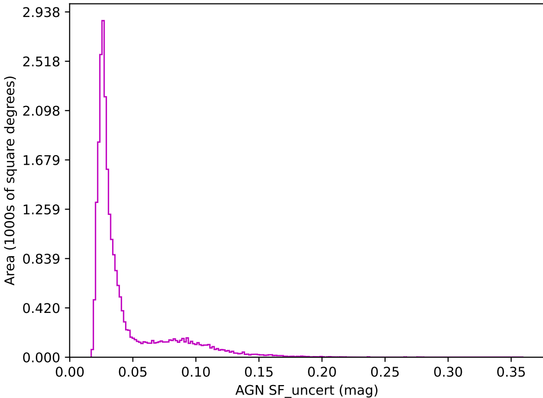
weather_cloudso31v3.4_10yrs z band: AGN SF_uncert
