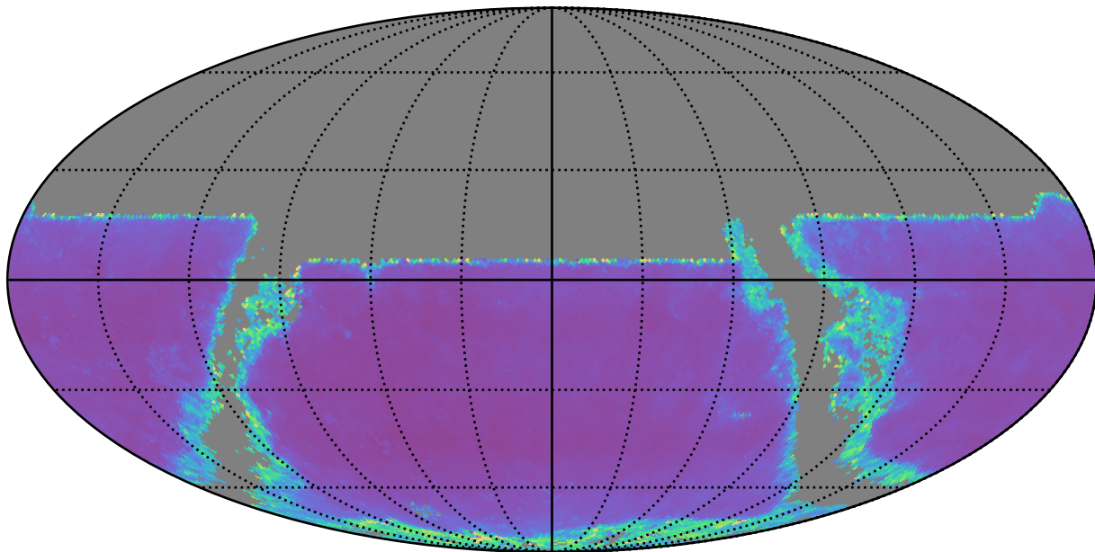
weather_cloudso31v3.4_10yrs y band: AGN SF_uncert
