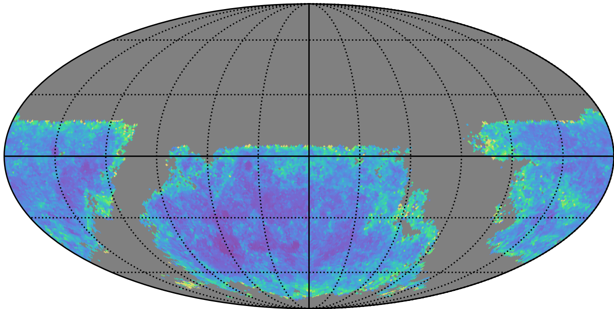
weather_cloudso31v3.4_10yrs u band: AGN SF_uncert
