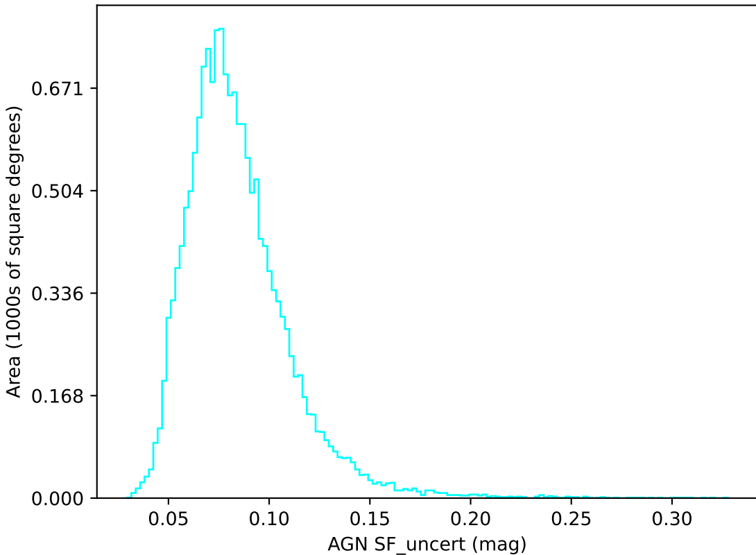
weather_cloudso31v3.4_10yrs u band: AGN SF_uncert
