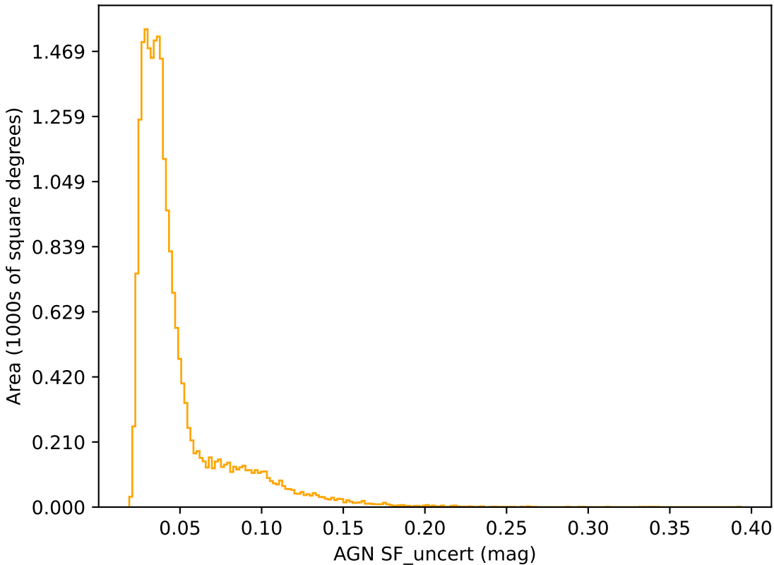
weather_cloudso31v3.4_10yrs r band: AGN SF_uncert
