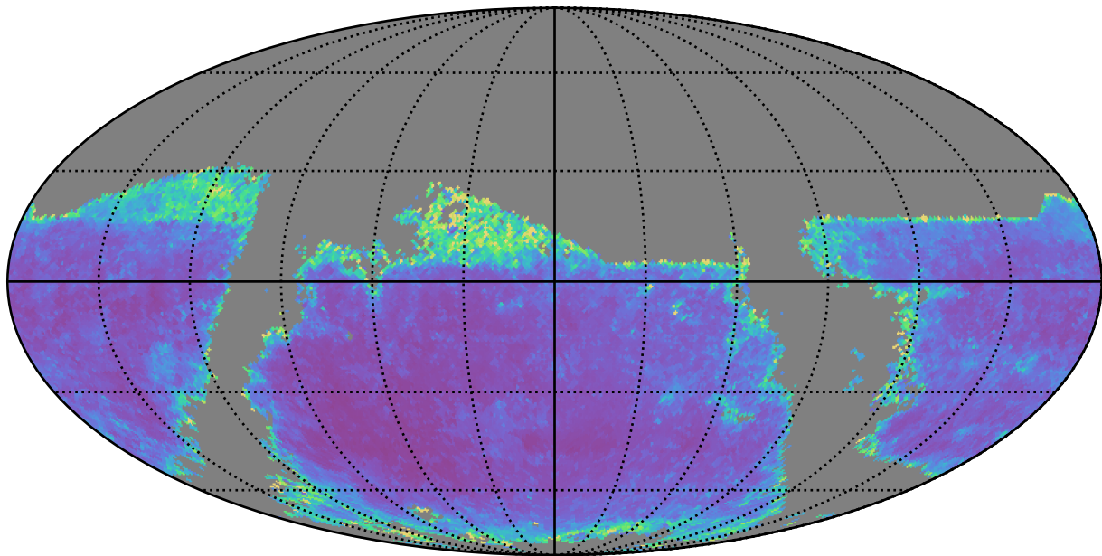
weather_cloudso31v3.4_10yrs g band: AGN SF_uncert
