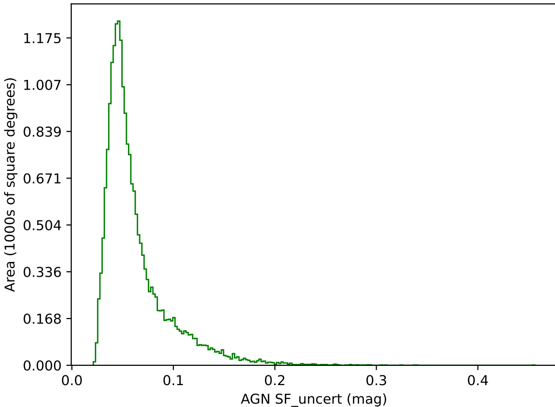
weather_cloudso31v3.4_10yrs g band: AGN SF_uncert
