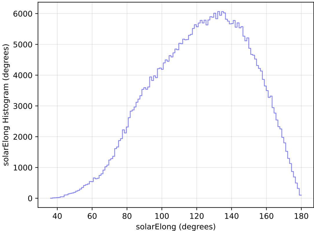
weather_cloudso31v3.4_10yrs WFD y band: solarElong Histogram
