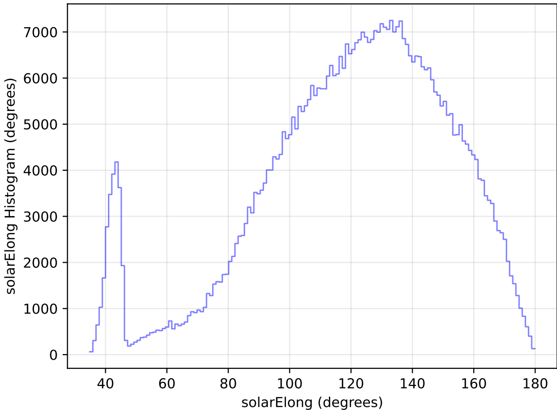
weather_cloudso31v3.4_10yrs WFD i band: solarElong Histogram
