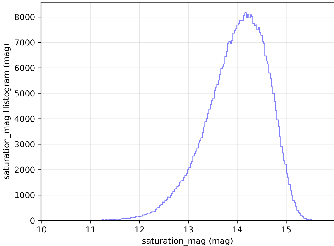
weather_cloudso31v3.4_10yrs WFD z band: saturation_mag Histogram
