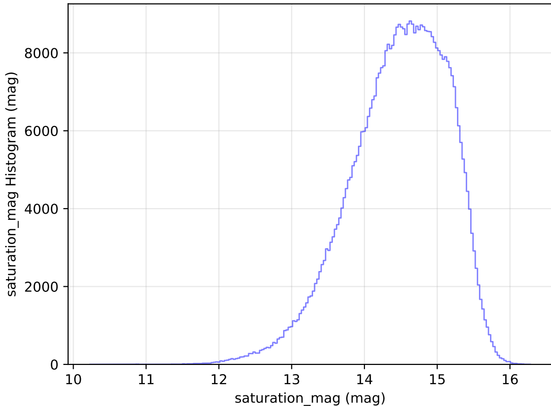
weather_cloudso31v3.4_10yrs WFD r band: saturation_mag Histogram
