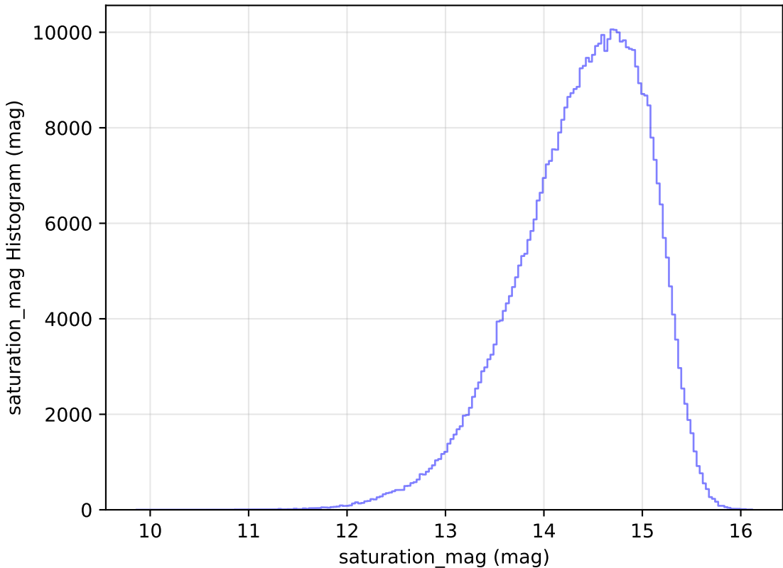
weather_cloudso31v3.4_10yrs WFD i band: saturation_mag Histogram
