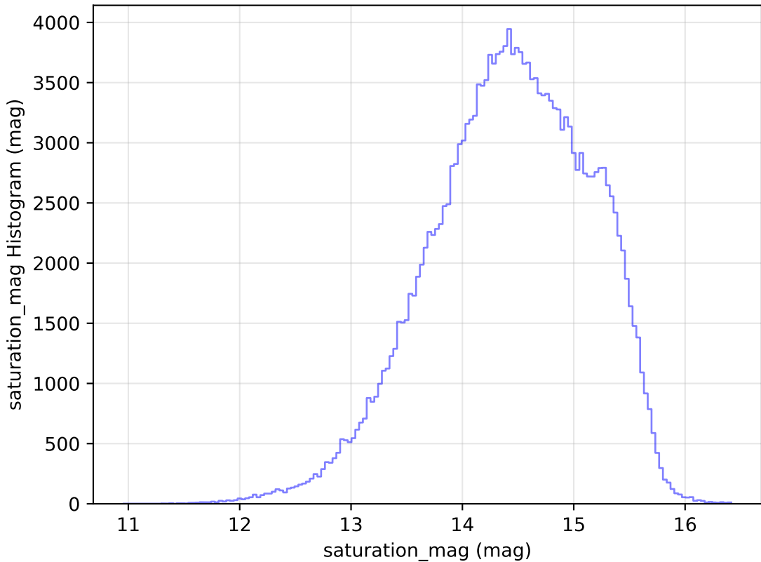
weather_cloudso31v3.4_10yrs WFD g band: saturation_mag Histogram
