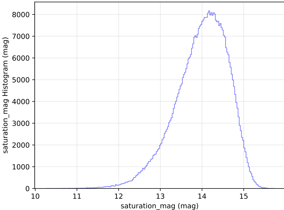
weather_cloudso31v3.4_10yrs All sky z band: saturation_mag Histogram
