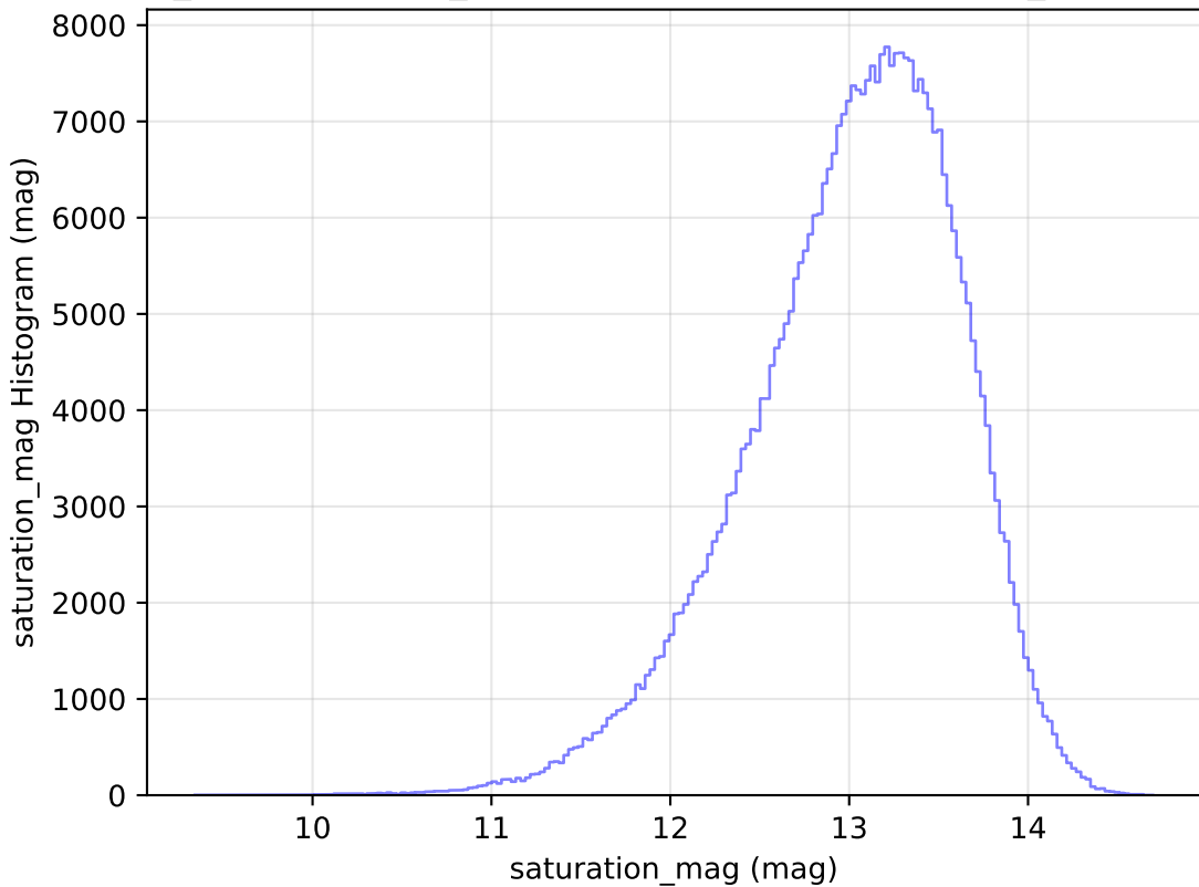
weather_cloudso31v3.4_10yrs All sky y band: saturation_mag Histogram
