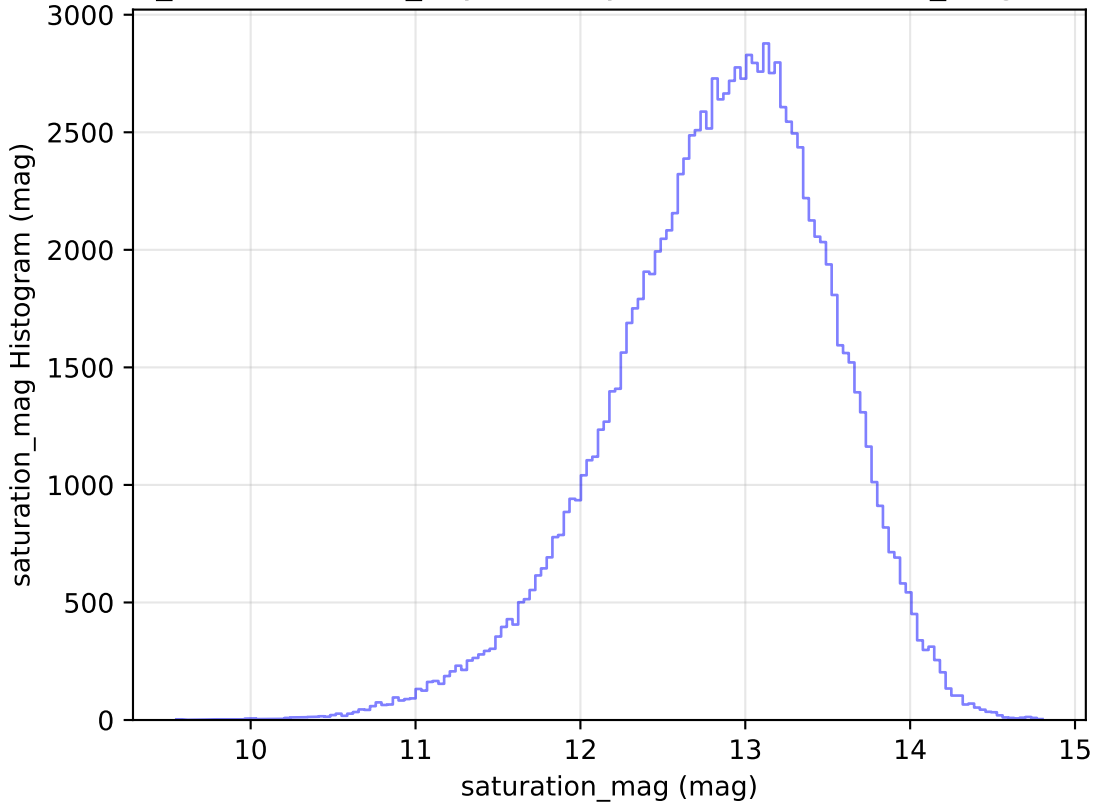
weather_cloudso31v3.4_10yrs All sky u band: saturation_mag Histogram
