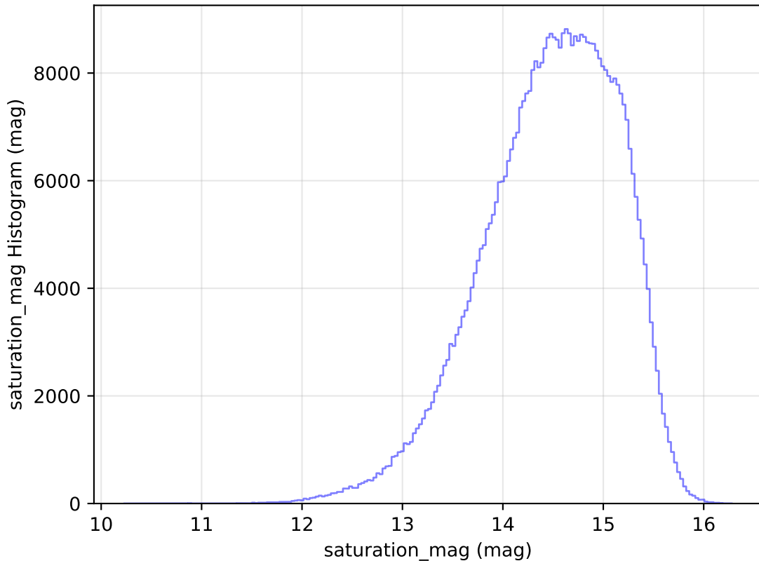
weather_cloudso31v3.4_10yrs All sky r band: saturation_mag Histogram
