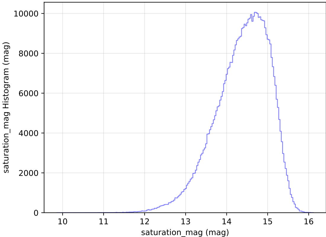
weather_cloudso31v3.4_10yrs All sky i band: saturation_mag Histogram
