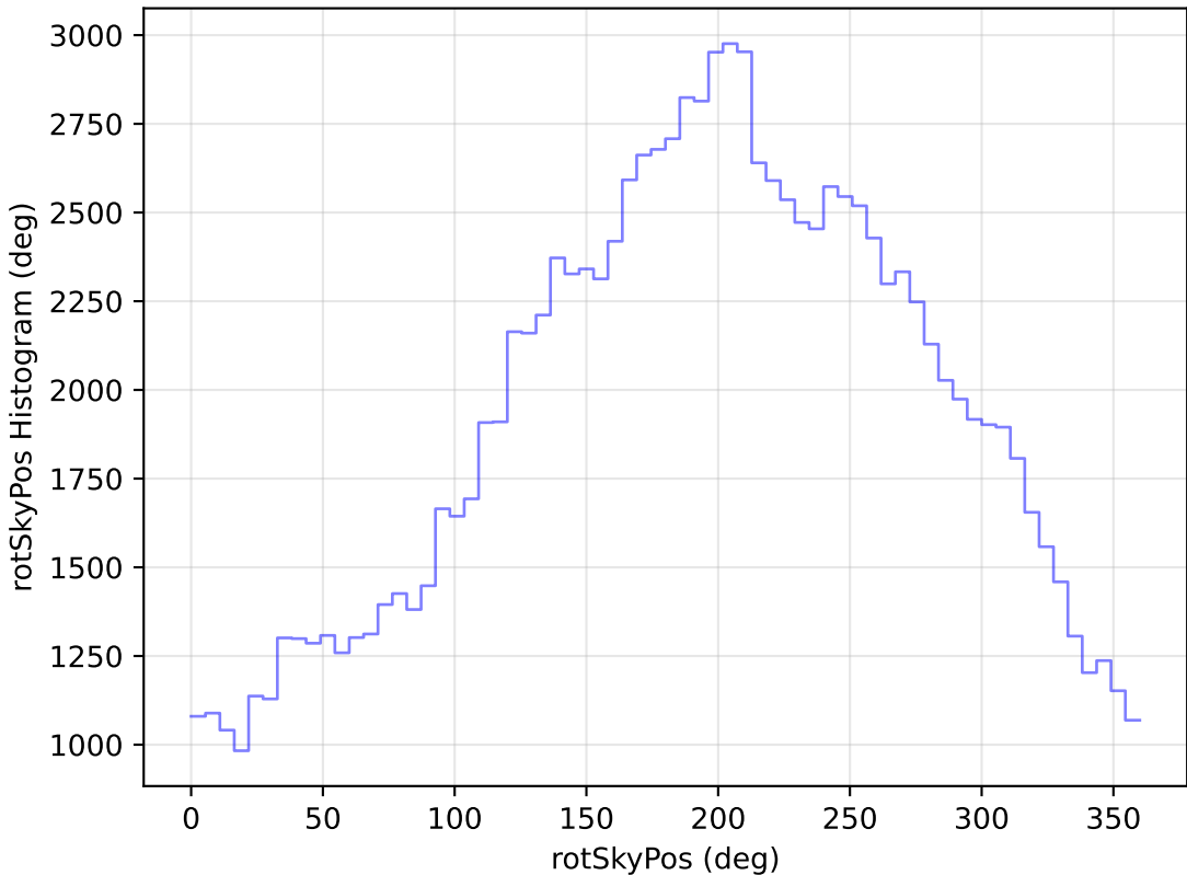
weather_cloudso31v3.4_10yrs WFD u band: rotSkyPos Histogram
