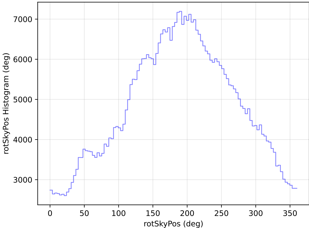
weather_cloudso31v3.4_10yrs WFD r band: rotSkyPos Histogram
