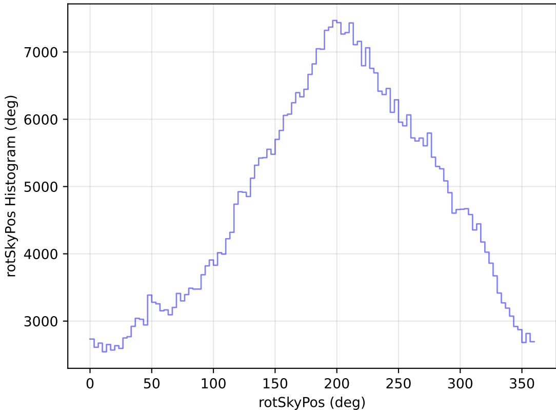
weather_cloudso31v3.4_10yrs WFD i band: rotSkyPos Histogram
