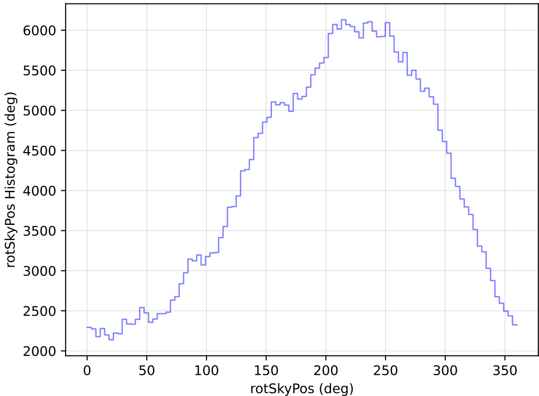
weather_cloudso31v3.4_10yrs All sky y band: rotSkyPos Histogram
