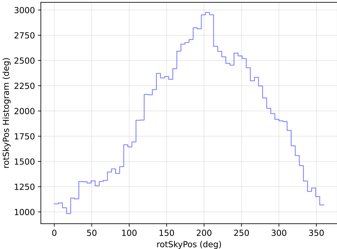
weather_cloudso31v3.4_10yrs All sky u band: rotSkyPos Histogram
