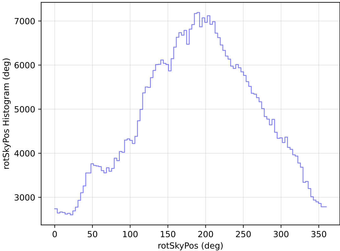
weather_cloudso31v3.4_10yrs All sky r band: rotSkyPos Histogram
