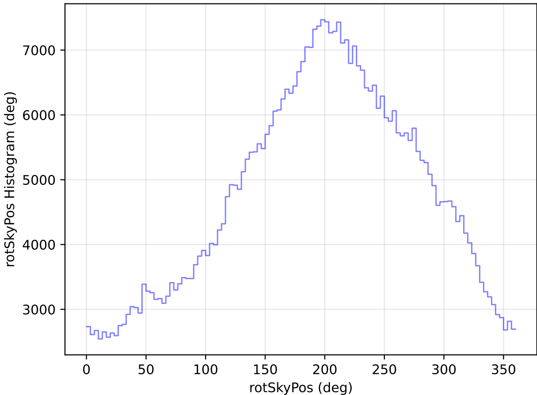
weather_cloudso31v3.4_10yrs All sky i band: rotSkyPos Histogram
