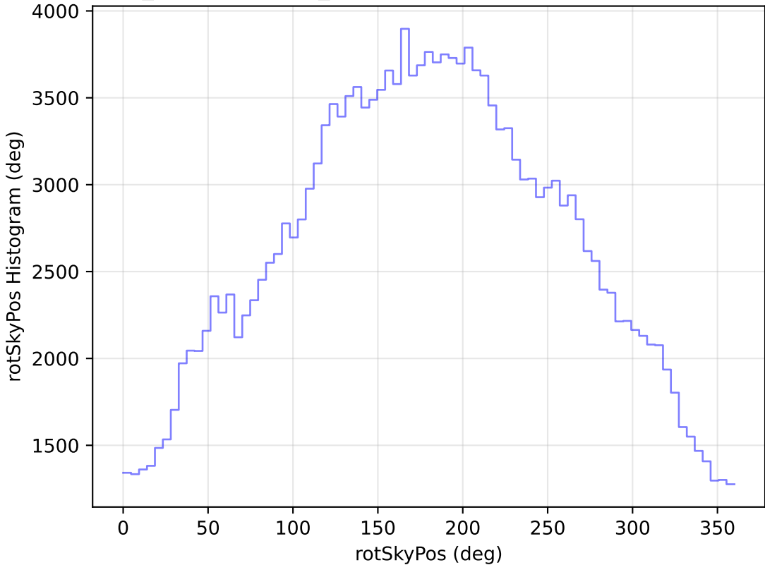
weather_cloudso31v3.4_10yrs All sky g band: rotSkyPos Histogram
