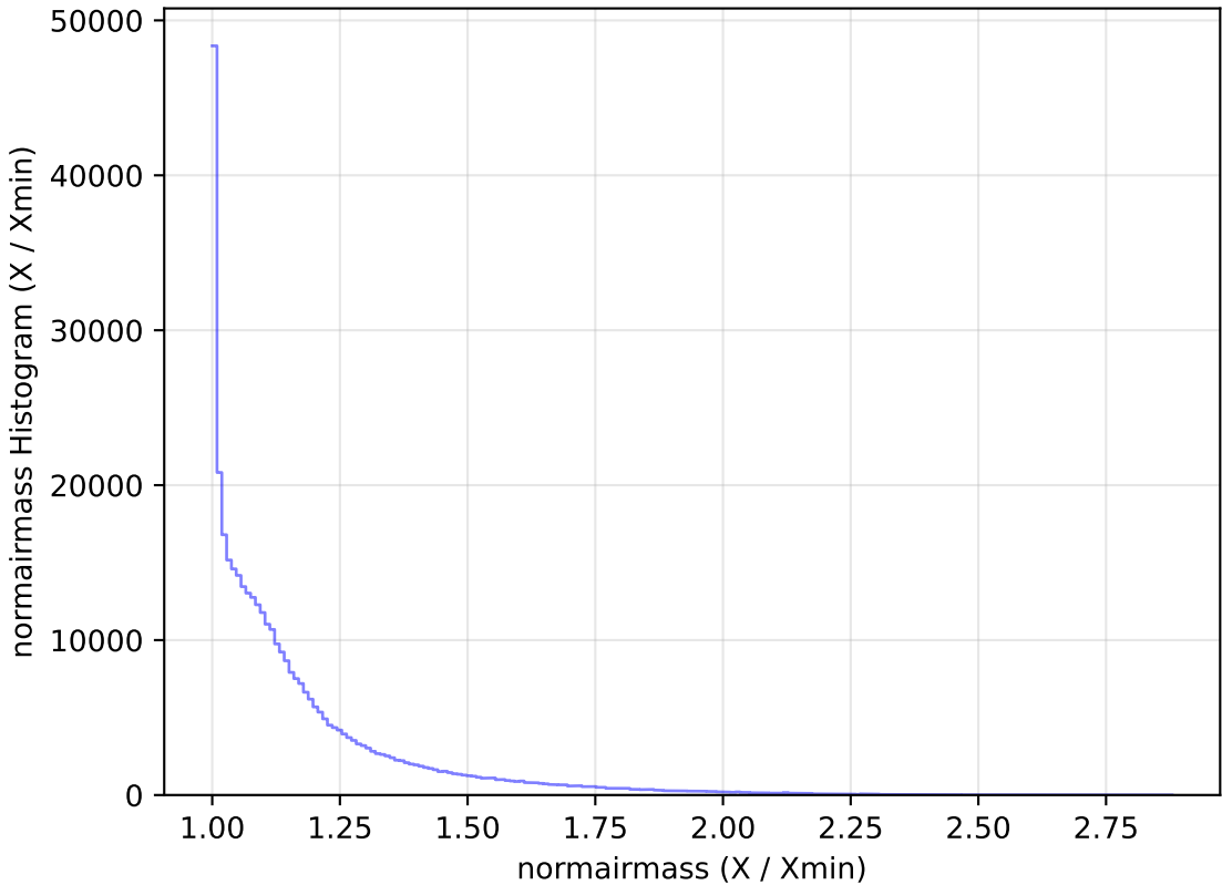
weather_cloudso31v3.4_10yrs All sky y band: normairmass Histogram
