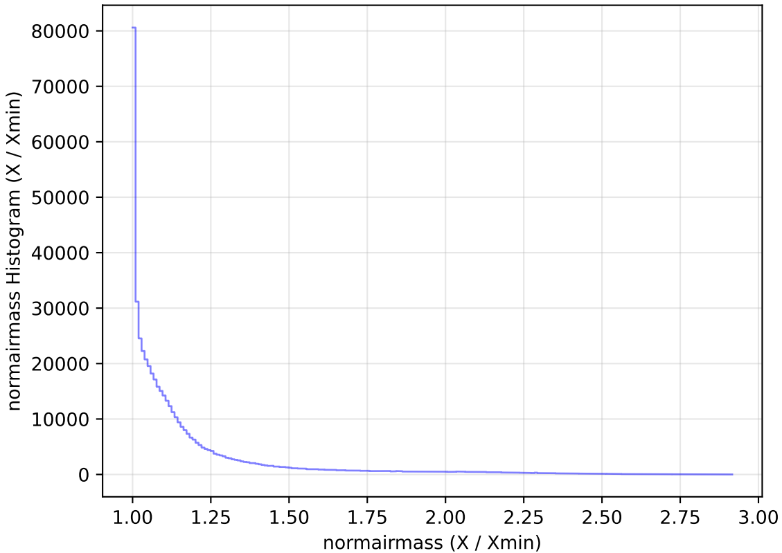
weather_cloudso31v3.4_10yrs All sky i band: normairmass Histogram
