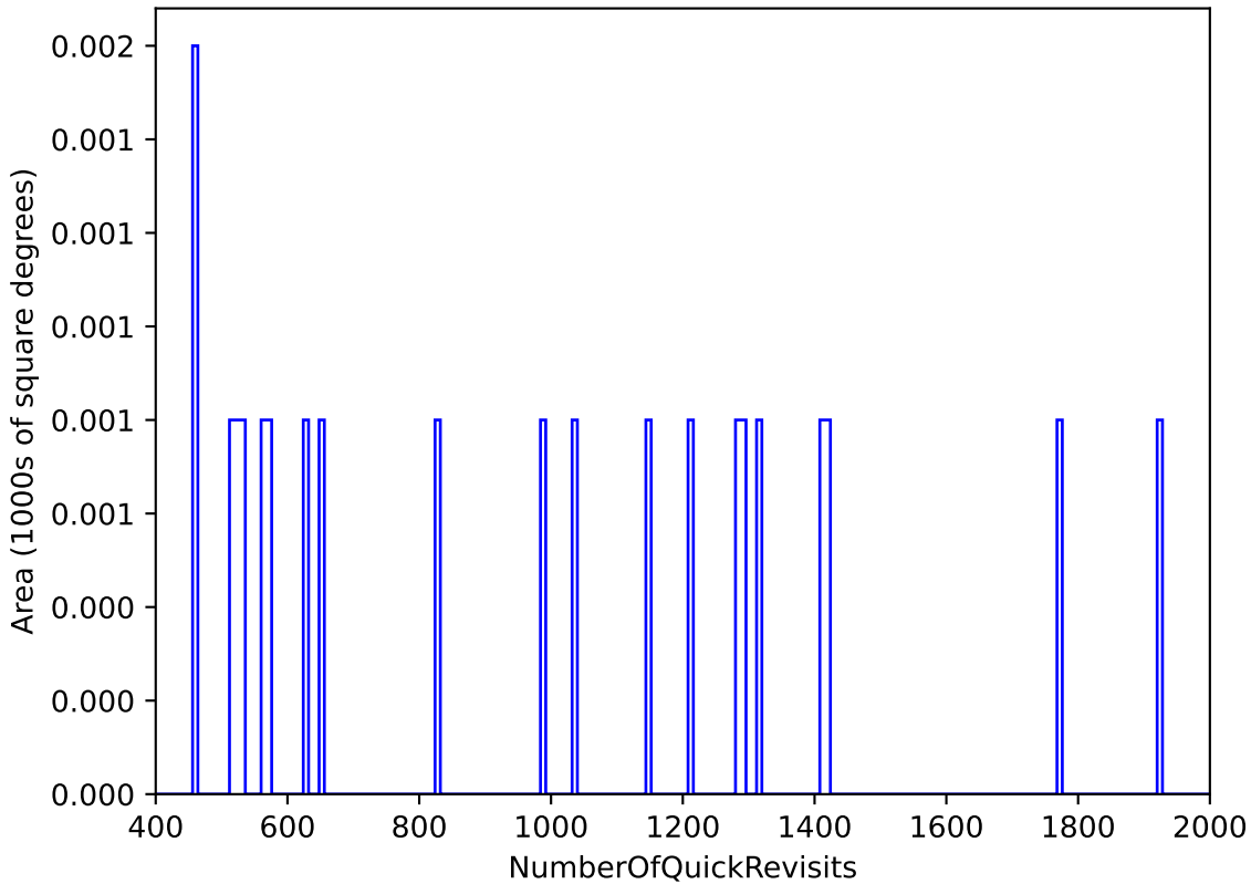
weather_cloudso31v3.4_10yrs WFD: NumberOfQuickRevisits
