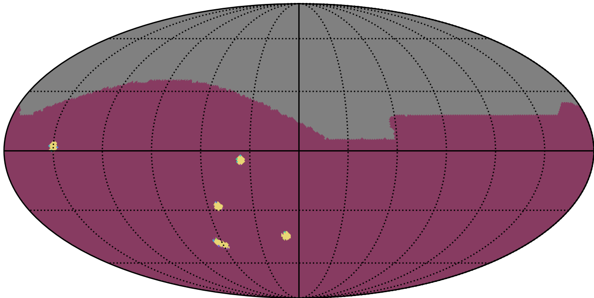
weather_cloudso31v3.4_10yrs All sky: NumberOfQuickRevisits
