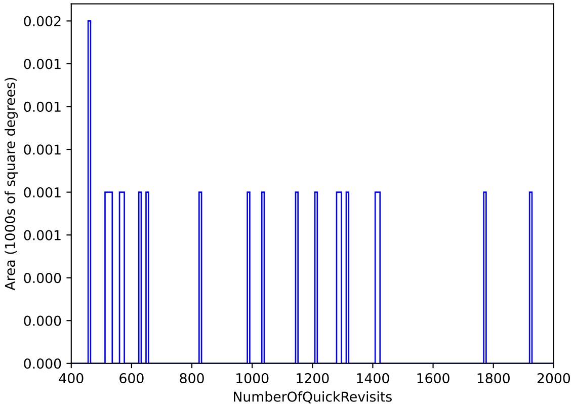
weather_cloudso31v3.4_10yrs All sky: NumberOfQuickRevisits
