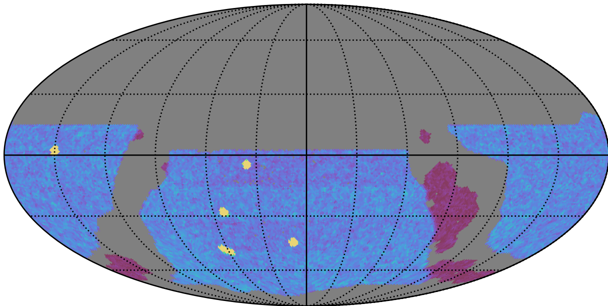
weather_cloudso31v3.4_10yrs WFD y band: NVisits
