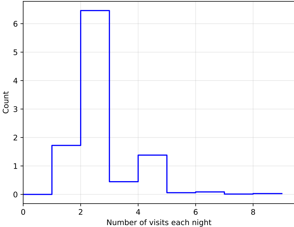
weather_cloudso31v3.4_10yrs All sky: NVisitsPerNight
