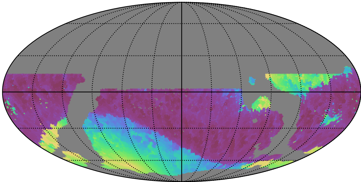
weather_cloudso31v3.4_10yrs WFD z band: Min solarElong
