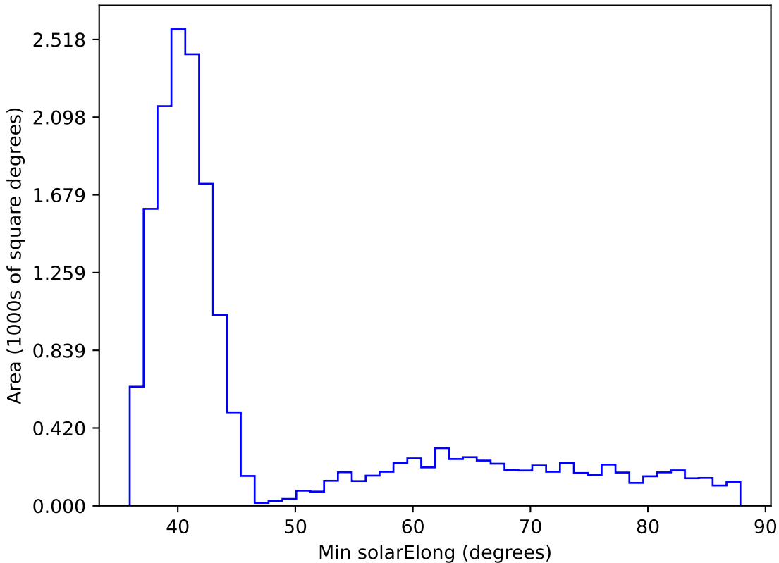
weather_cloudso31v3.4_10yrs WFD z band: Min solarElong
