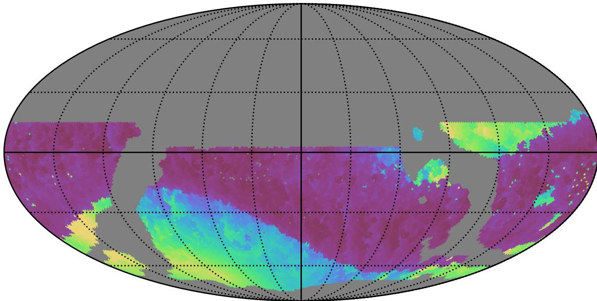
weather_cloudso31v3.4_10yrs WFD i band: Min solarElong
