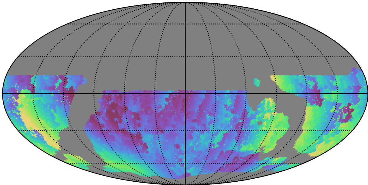
weather_cloudso31v3.4_10yrs WFD g band: Min solarElong
