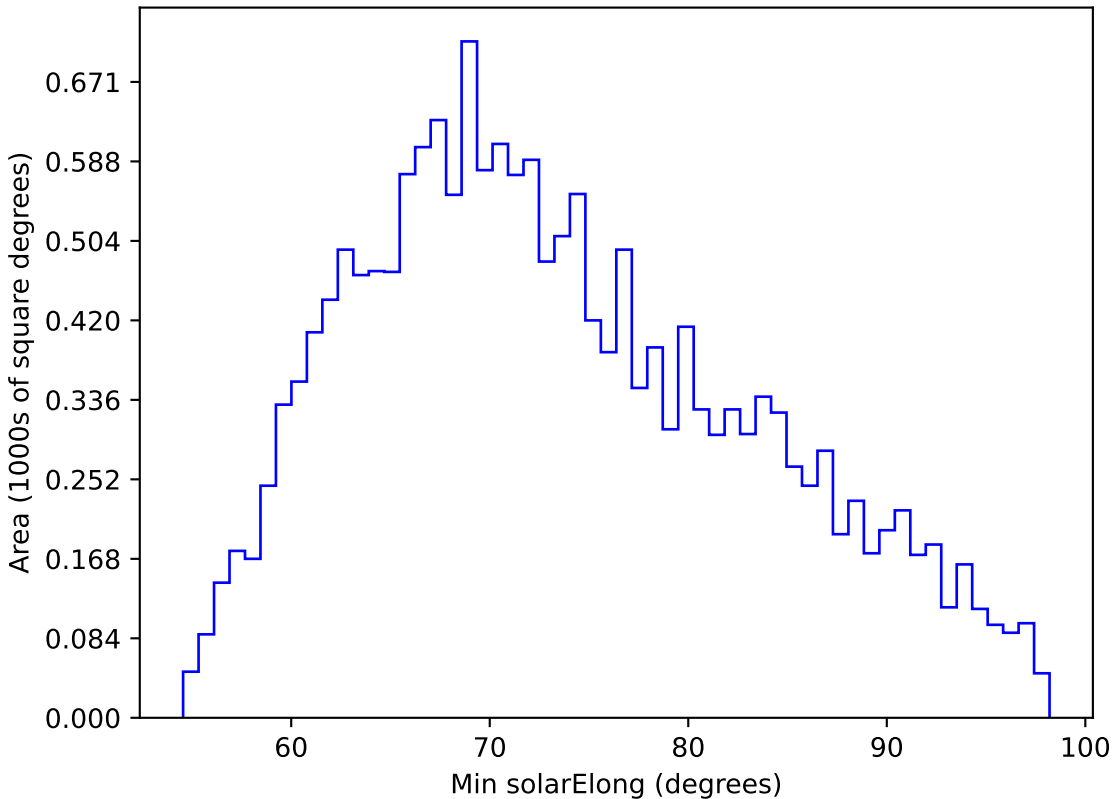
weather_cloudso31v3.4_10yrs WFD g band: Min solarElong
