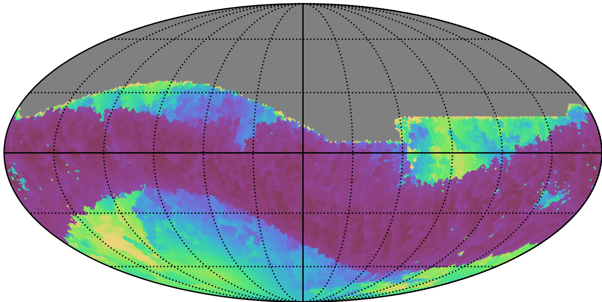
weather_cloudso31v3.4_10yrs All sky z band: Min solarElong
