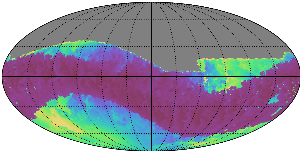
weather_cloudso31v3.4_10yrs All sky i band: Min solarElong
