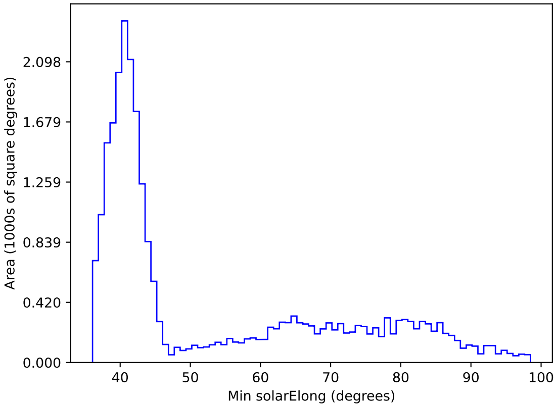
weather_cloudso31v3.4_10yrs All sky i band: Min solarElong
