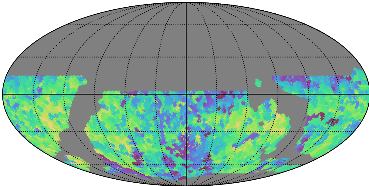
weather_cloudso31v3.4_10yrs WFD y band: Min saturation_mag
