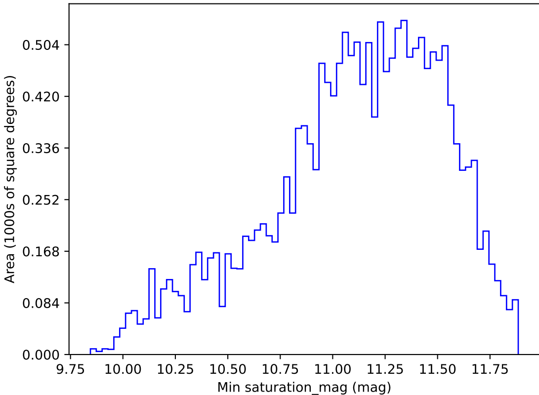
weather_cloudso31v3.4_10yrs WFD y band: Min saturation_mag
