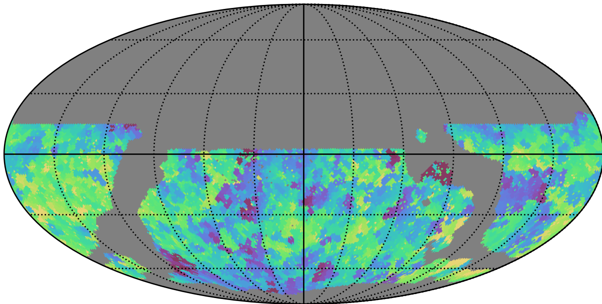
weather_cloudso31v3.4_10yrs WFD u band: Min saturation_mag
